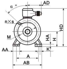
IMB35
