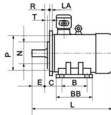
IMB35
